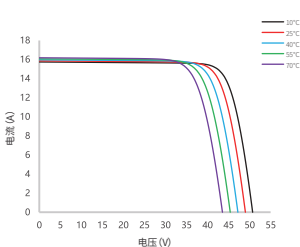
电流-电压曲线 SSA-66HD-610N
