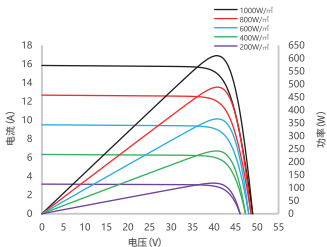
电流/功率-电压曲线 SSA-66HD-610N
